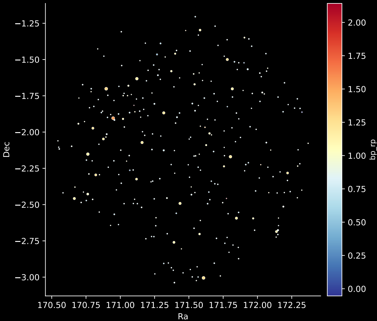
GALAH DR4 Field: [1096] Stars: 283
