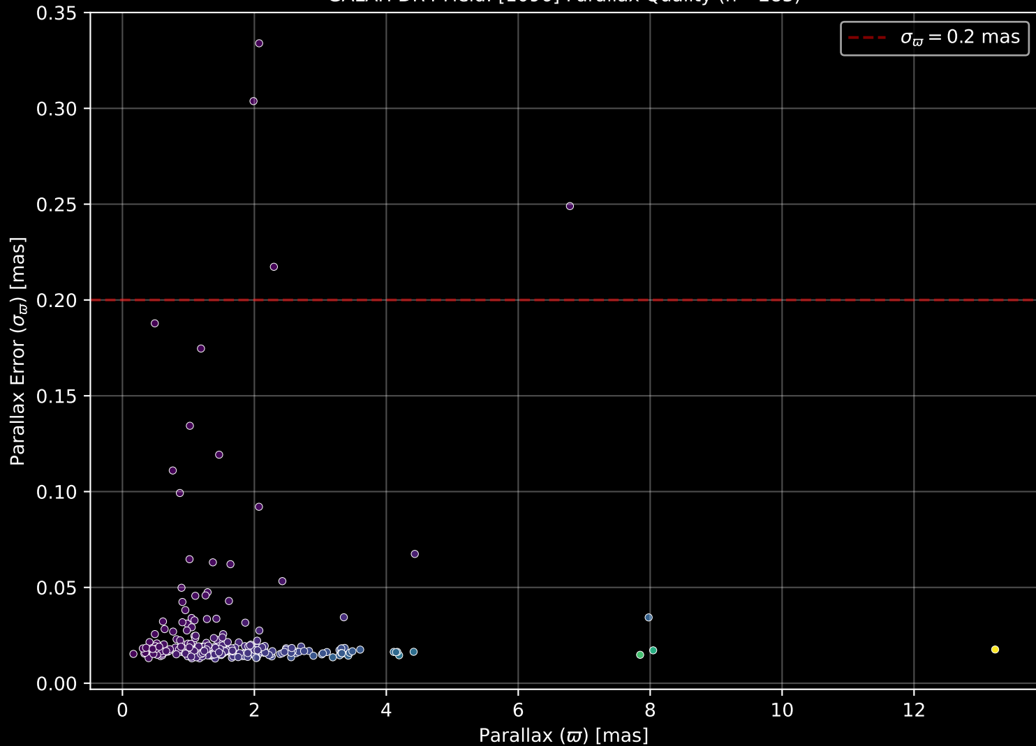
GALAH DR4 Field: [1096] Parallax Quality (n= 283)
