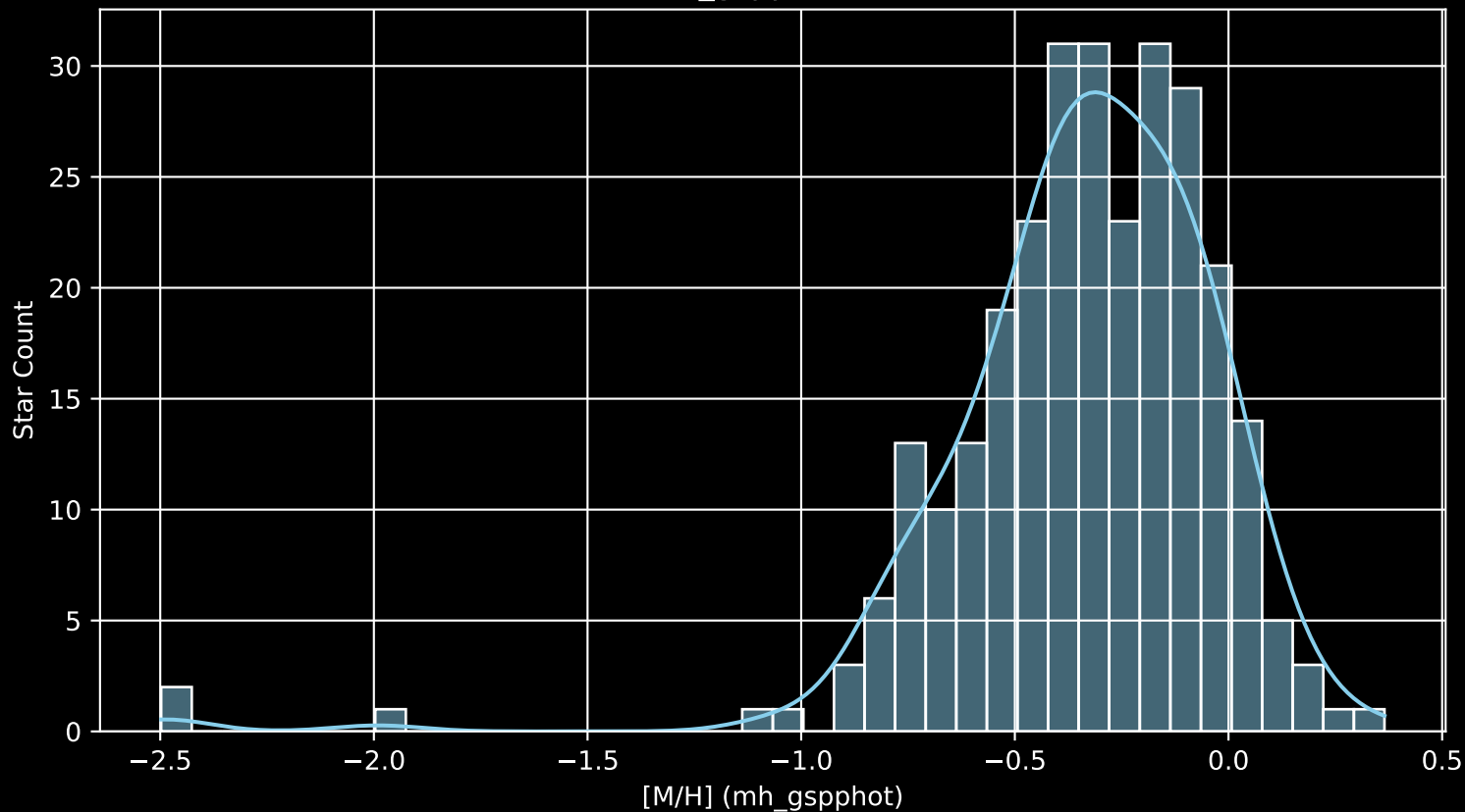
GALAH DR4 Field: [1096] [M/H] (mh_gspphot) (n= 282)
