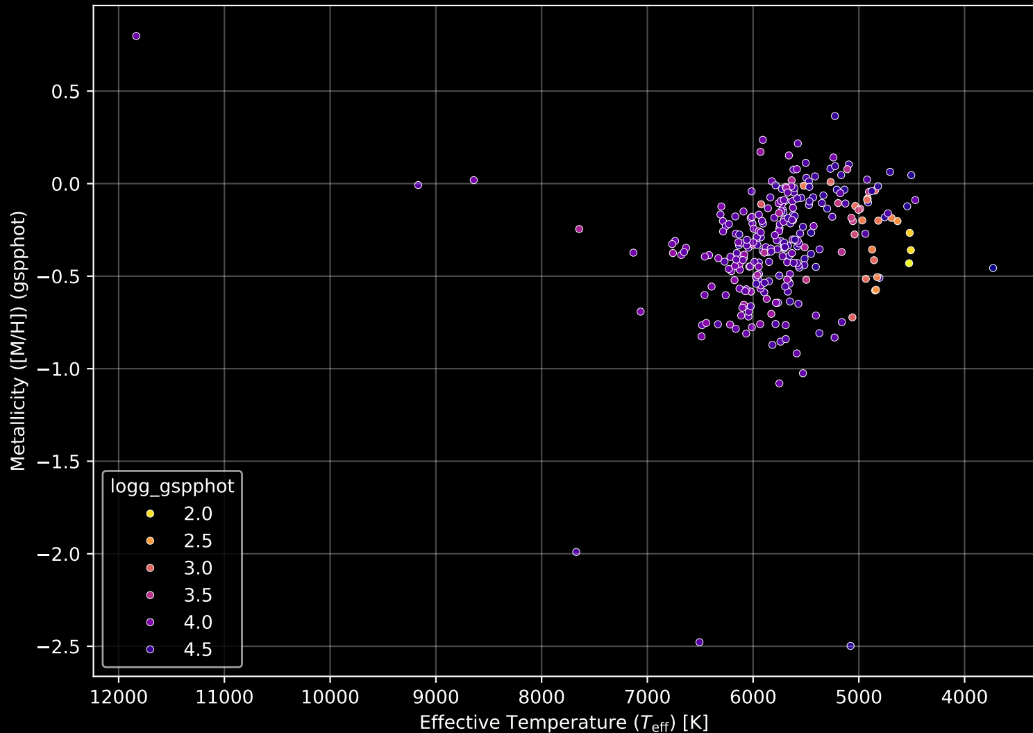
GALAH DR4 Field: [1096] Stellar Population Parameters (n= 283)
