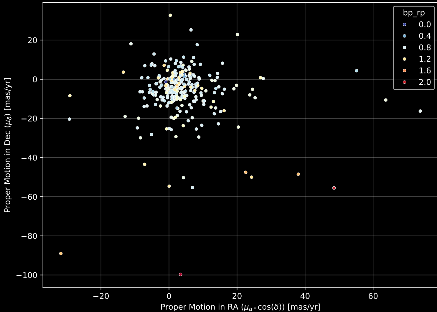
GALAH DR4 Field: [1096] Proper Motion Diagram (n= 283)
